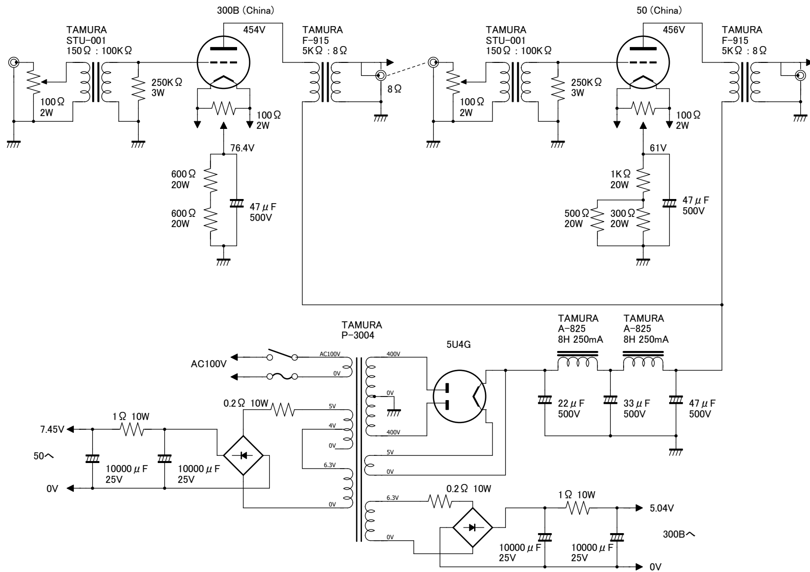
300Bシングルドライブ50シングルコンパチブルパワーアンプ 佐久間駿設計・製作 2015年8月
