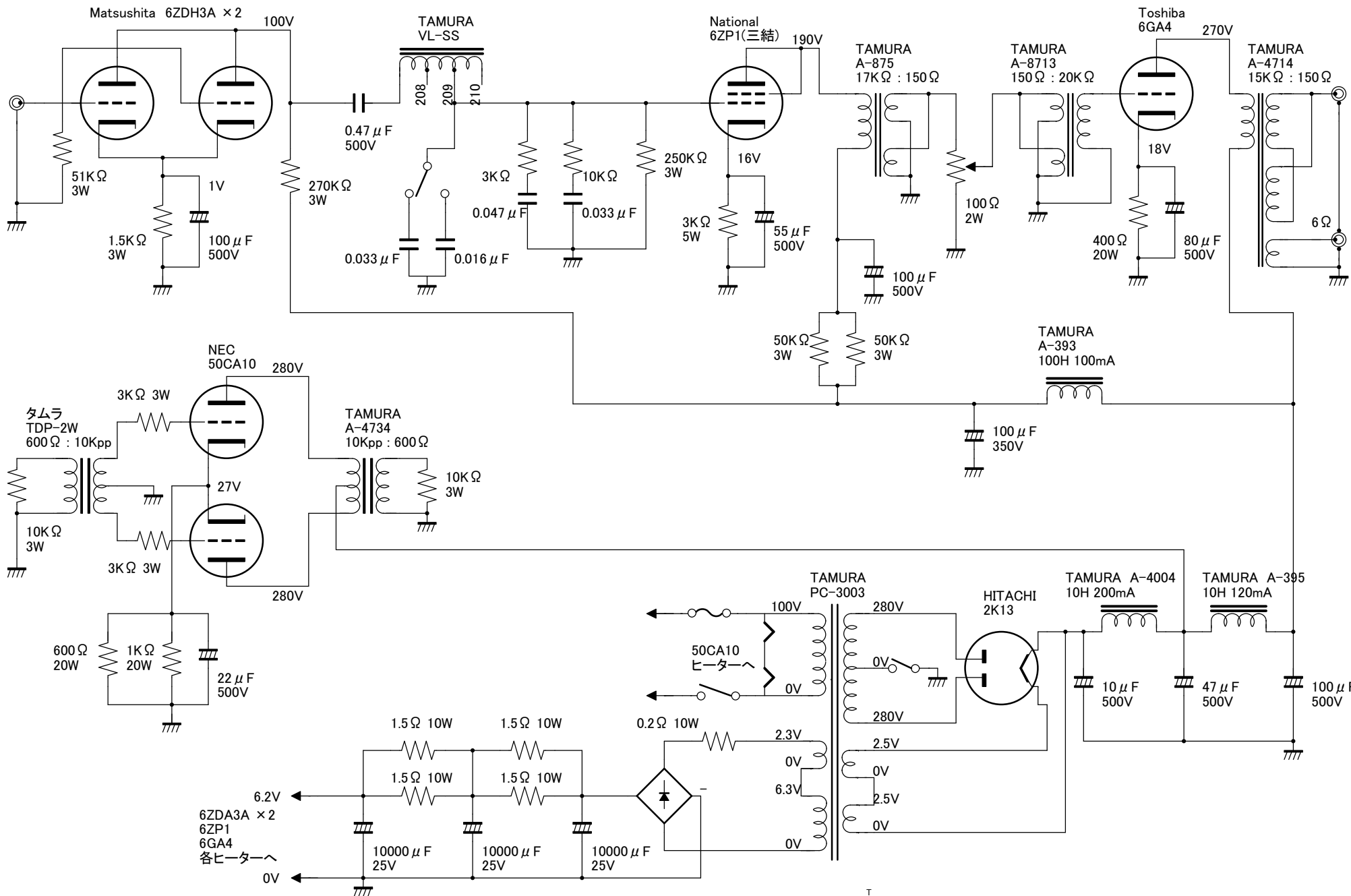
T 6GA4POWER_TRANS
